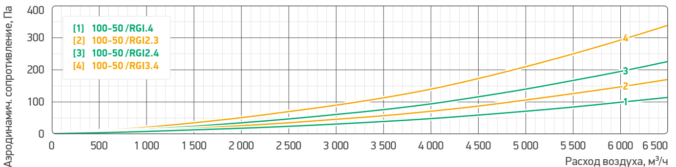
Аэродинамические характеристики секций теплоутилизатора гликолевого 100-50 /RGI
