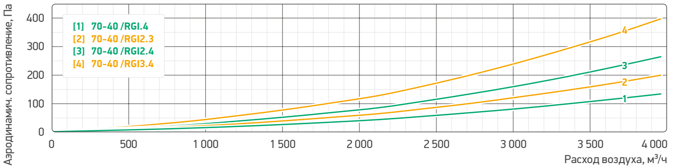
Аэродинамические характеристики секций теплоутилизатора гликолевого 80-50 /RGI
