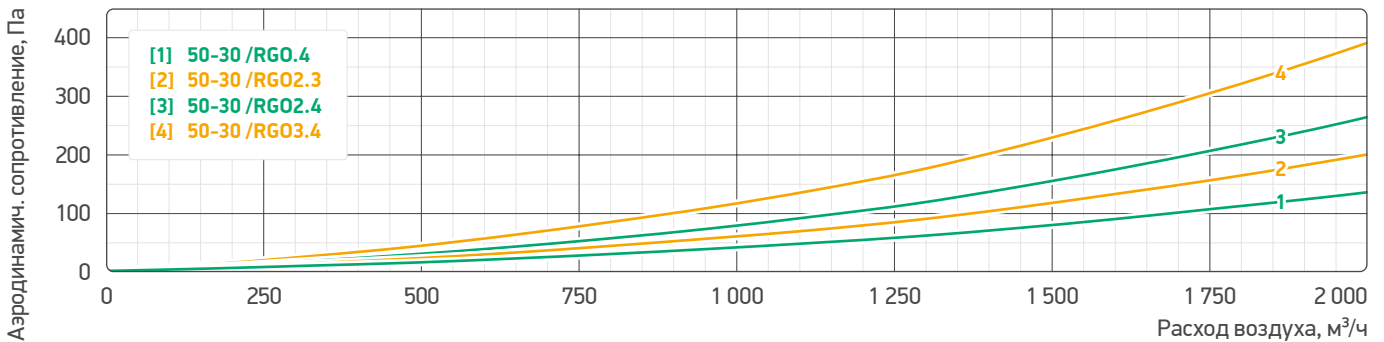
Аэродинамические характеристики секций теплоутилизатора гликолевого 60-30 /RGO
