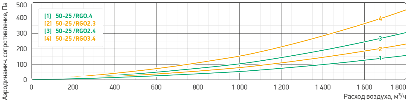
Аэродинамические характеристики секций теплоутилизатора гликолевого 50-30 /RGO
