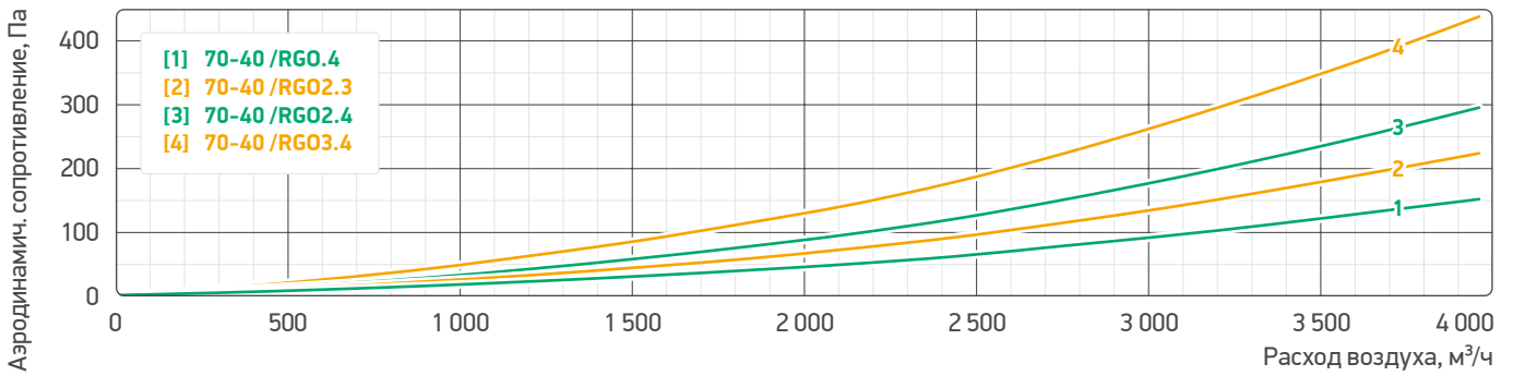
Аэродинамические характеристики секций теплоутилизатора гликолевого 80-50 /RGO
