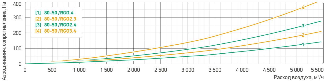
Аэродинамические характеристики секций теплоутилизатора гликолевого 90-50 /RGO
