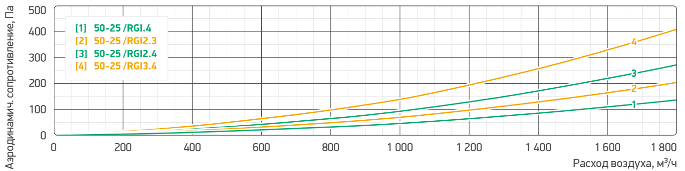
Аэродинамические характеристики секций теплоутилизатора гликолевого 50-30 /RGI
