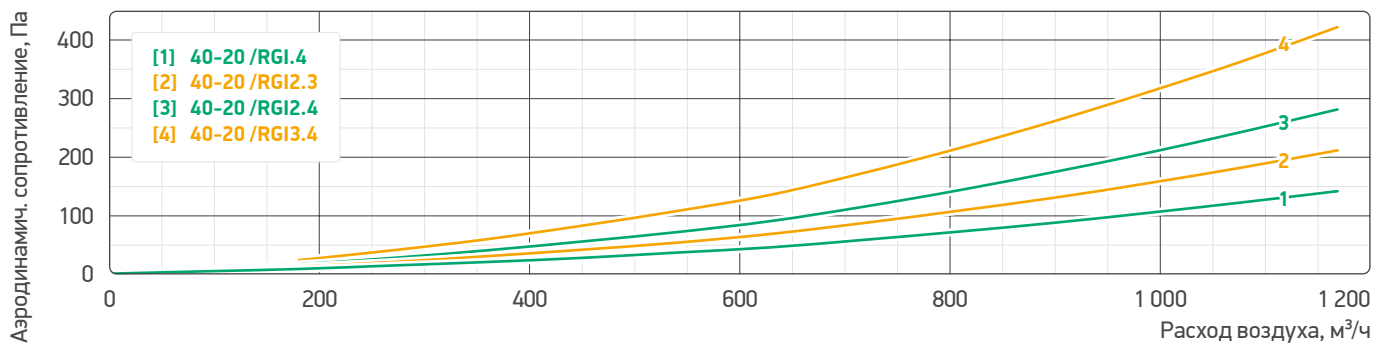
Аэродинамические характеристики секций теплоутилизатора гликолевого 50-25 /RGI
