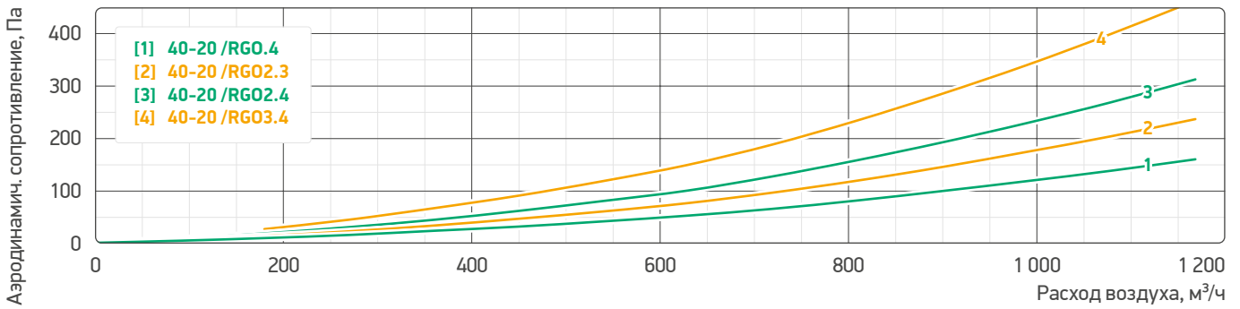
Аэродинамические характеристики секций теплоутилизатора гликолевого 50-25 /RGO
