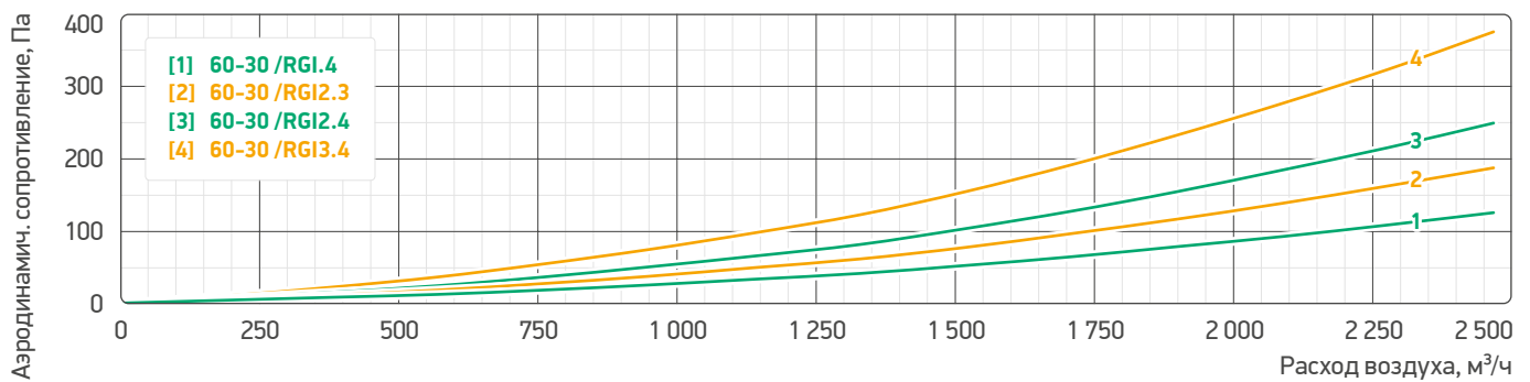
Аэродинамические характеристики секций теплоутилизатора гликолевого 60-30 /RGI
