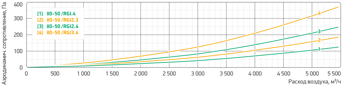
Аэродинамические характеристики секций теплоутилизатора гликолевого 90-50 /RGI
