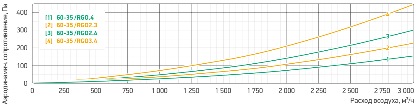
Аэродинамические характеристики секций теплоутилизатора гликолевого 60-35 /RGO
