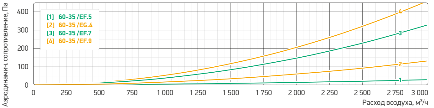
Аэродинамические характеристики фильтров воздушных 70-40 /EG, /EF
