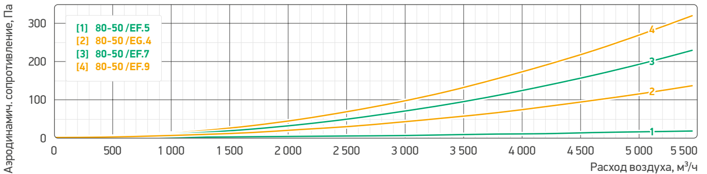
Аэродинамические характеристики фильтров воздушных 90-50 /EG, /EF
