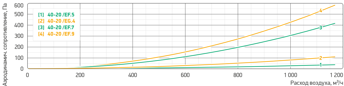
Аэродинамические характеристики фильтров воздушных 50-25 /EG, /EF
