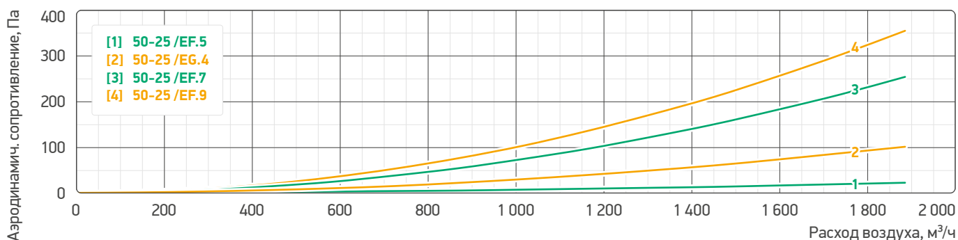
Аэродинамические характеристики фильтров воздушных 50-30 /EG, /EF
