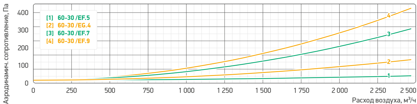
Аэродинамические характеристики фильтров воздушных 60-30 /EG, /EF
