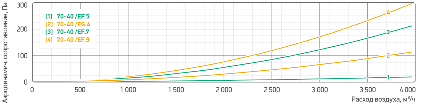
Аэродинамические характеристики фильтров воздушных 80-50 /EG, /EF
