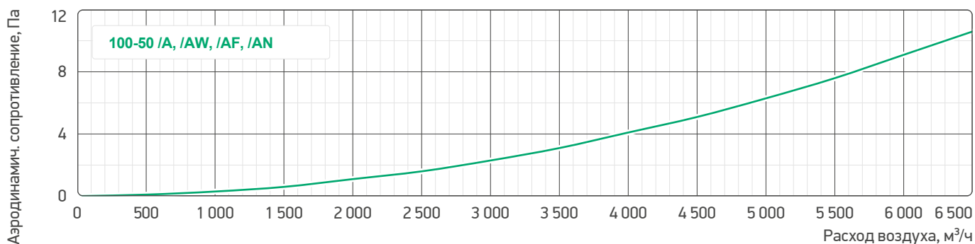
Гр. 9. Аэродинамические характеристики клапанов воздушных 100-50 /A
