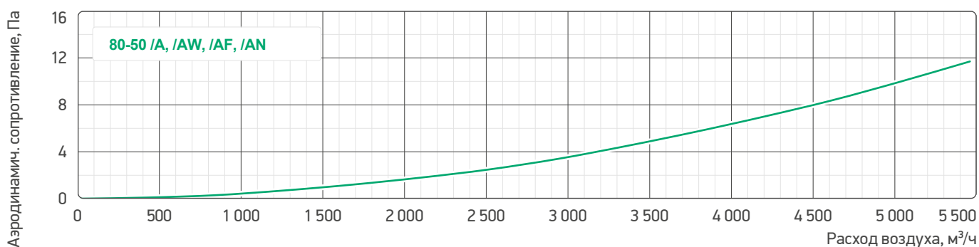
Гр. 8. Аэродинамические характеристики клапанов воздушных 90-50 /A
