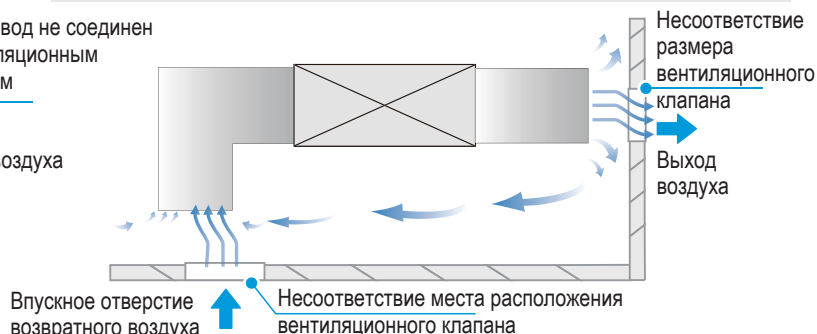
Несоответствие размера и места расположения вентиляционного клапана
