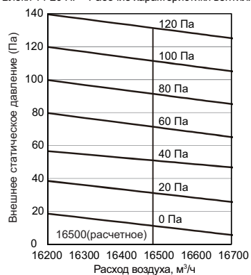
Блоки 14-20 НР - Рабочие характеристики вентилятора
