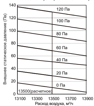
12 НР - Рабочие характеристики вентилятора
